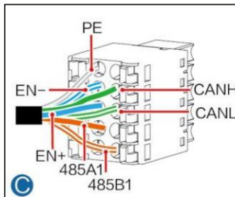
Batterie B connexion
