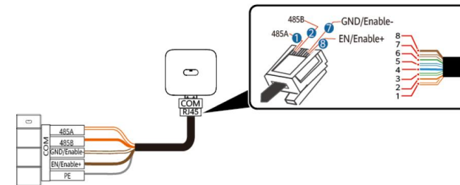
SUN2000-M1 et SUN2000-MB0
