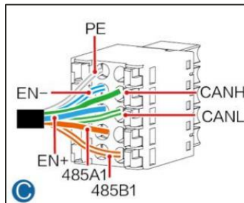
Batterie A connexion
