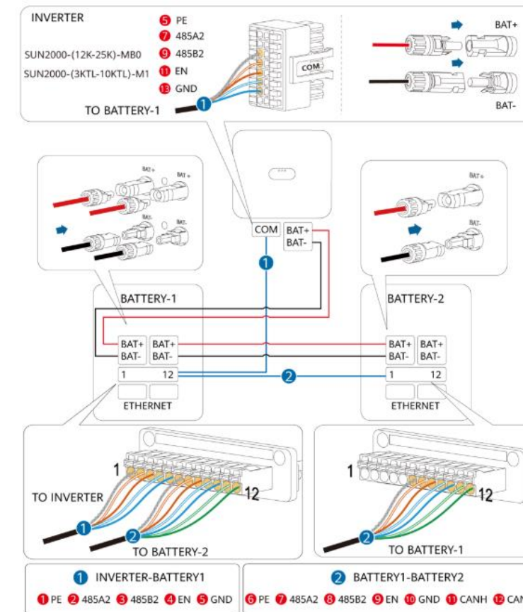
SUN2000-M1 et SUN2000-MB0
